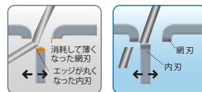
消耗した網刃と内刃 新しい網刃と内刃
